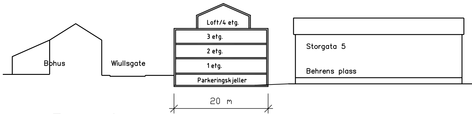
Terrengsnitt.
