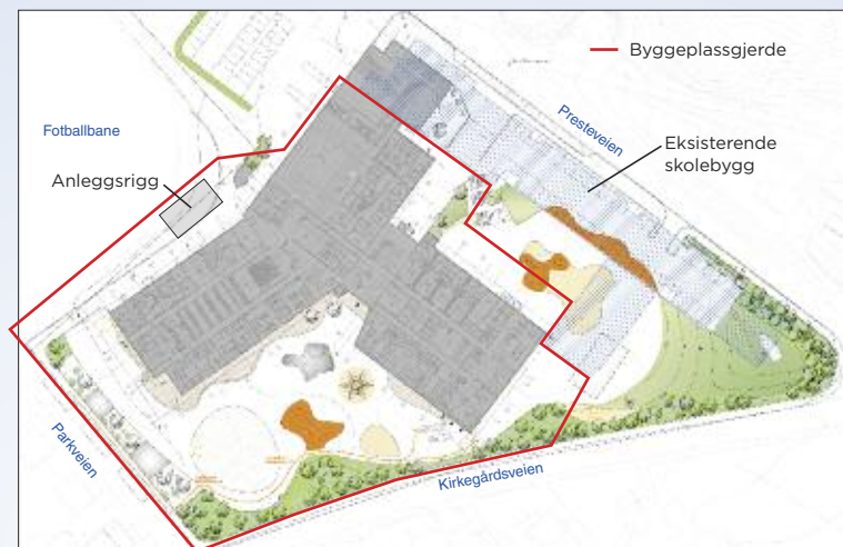
Oversiktstegning som viser byggeplass, gjerder, anleggsrigg og skoleområdet frem til 28.11.2011.
